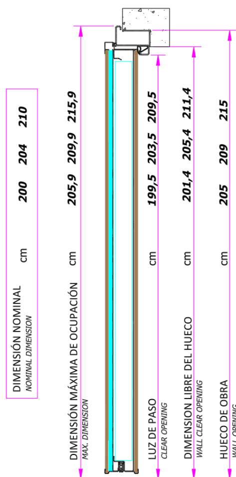
- SECCIÓN VERTICAL - VERTICAL SECTION
